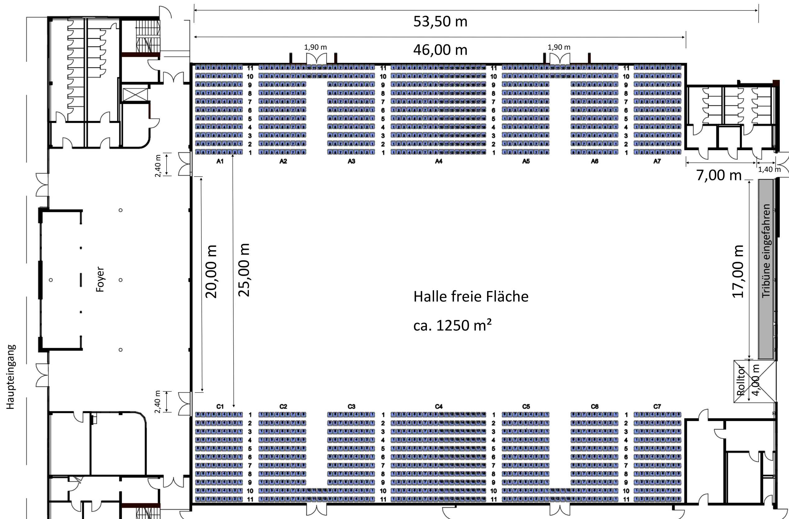
Sparkassen-Arena Jena - Halle 1 mit Tribünen Block A und C (schematische Darstellung)
